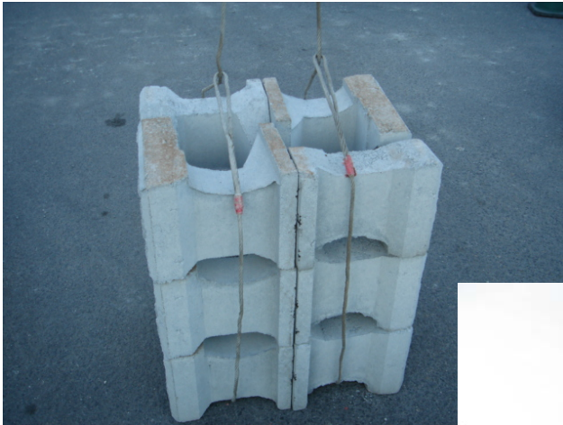
根石(B型)の 移動例です
